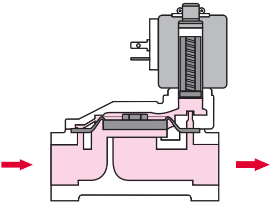
Bobina Energizada
