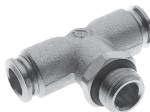
Racor Tee Horizontal - Giratorio
